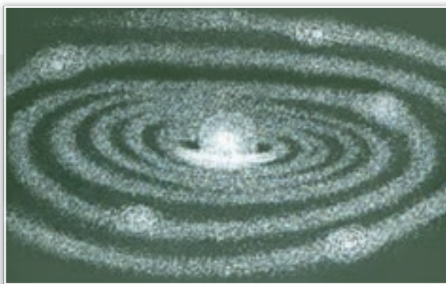
Планетарная модель атома. 1908—1909 гг.
