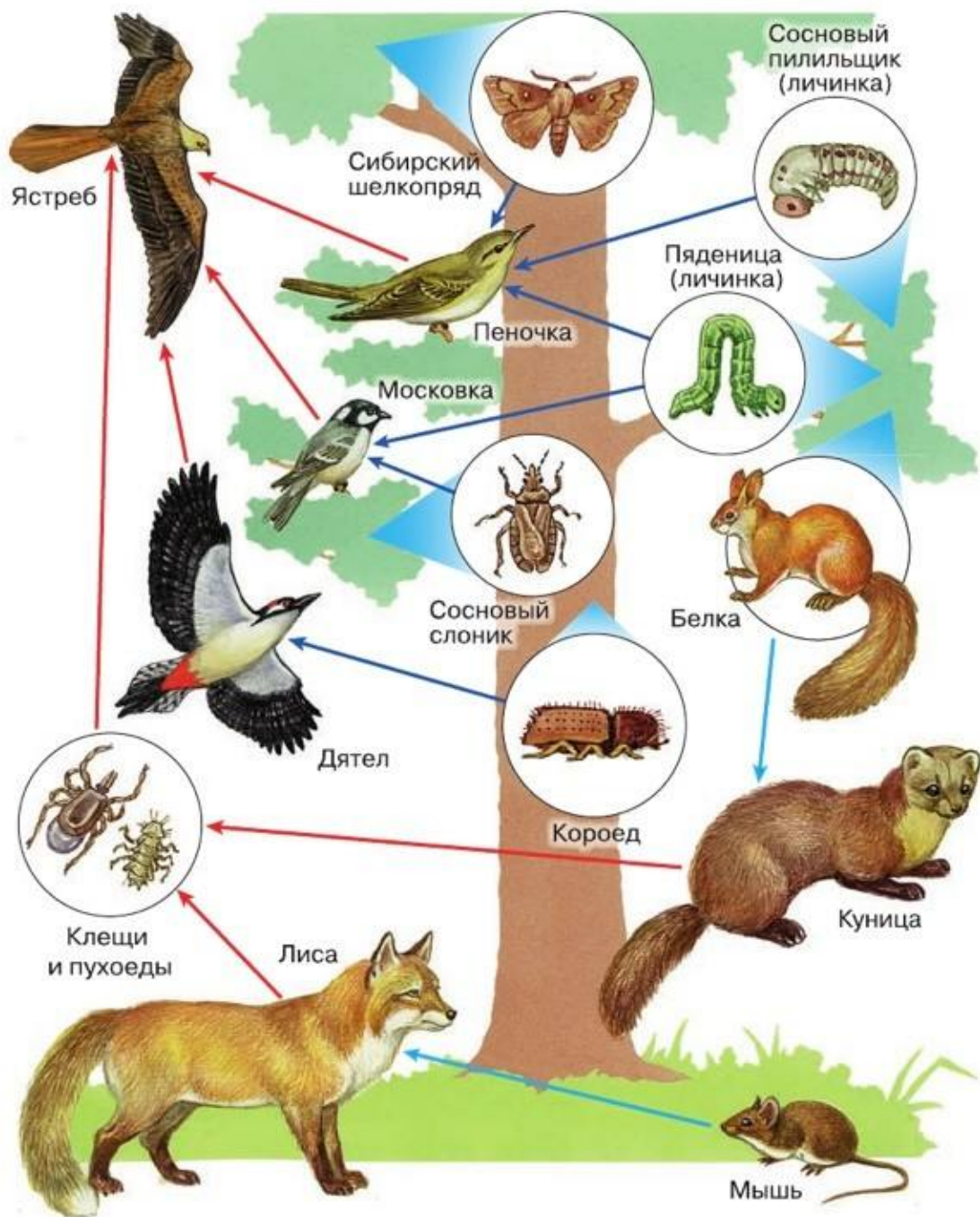
Рис. 101. Пример пищевой сети сообщества
