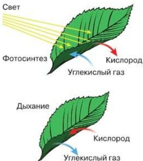
Рис. 53. Фотосинтез
