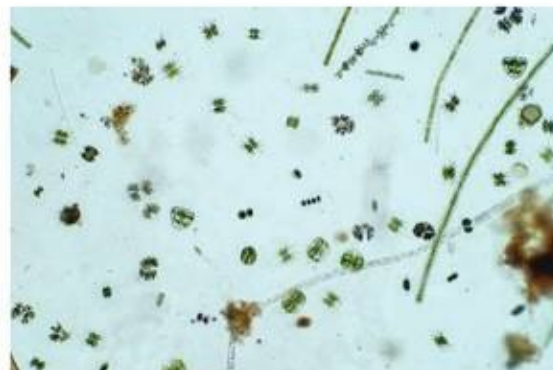
Рис. 80. Планктонные организмы
